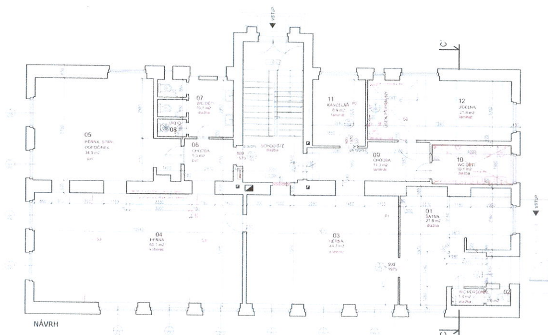
Obrázek č. 3. Půdorys stávající MŠ
